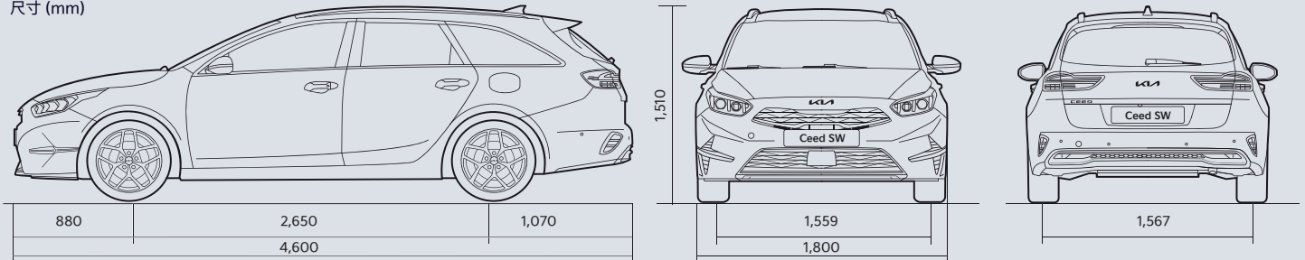
尺寸 (mm)
