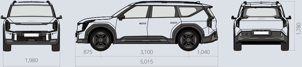
尺寸(mm) GT-line e-AWD 車型
